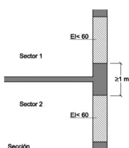
Figura 1.7 Encuentro forjado-fachada
